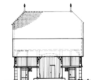
807 Elévation ouest 1:250
